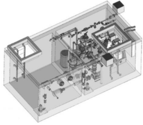
Şekil 226: Su deposu yerleşimi
