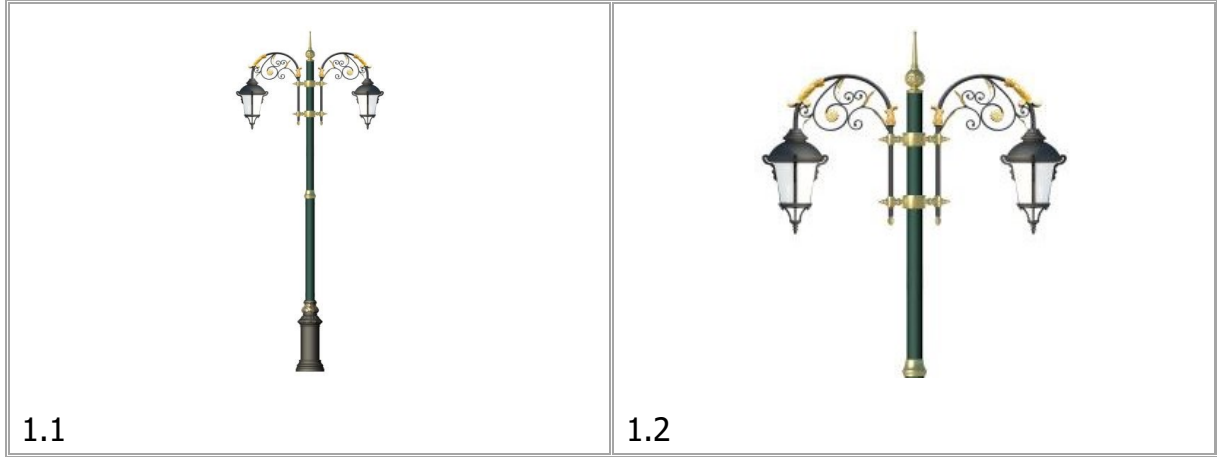
Şekil 79: Dış mekân aydınlatma direği
